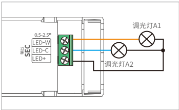
单地址双通道—每路最大输出总功率50%
