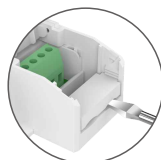
向外推线板的同时, 用工具撬即可拆下压线板。
