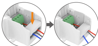
向下推压线板, 可固定住线。
