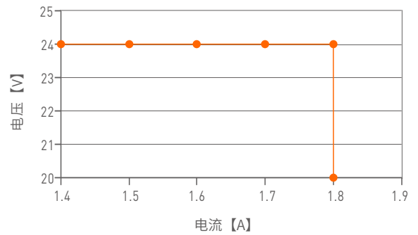
过载曲线
