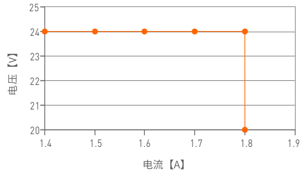
过载曲线
