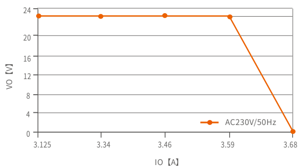
过载曲线
