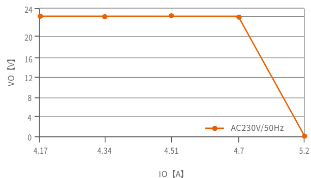
过载曲线
