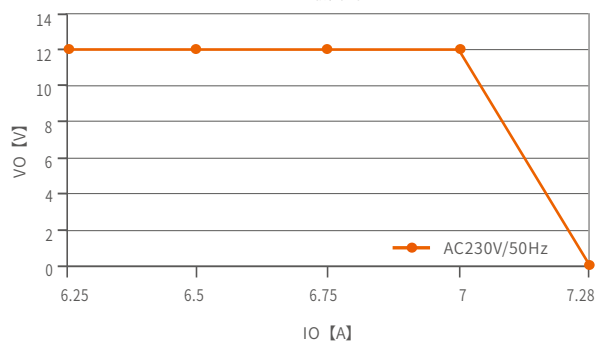
过载曲线
